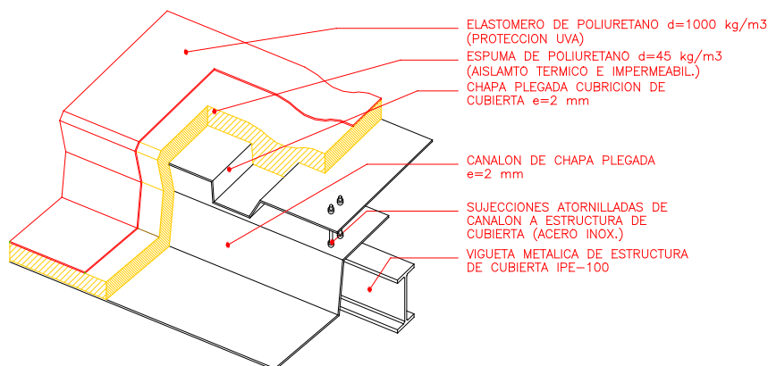
Proyección de poliuretano integrando las greclas
