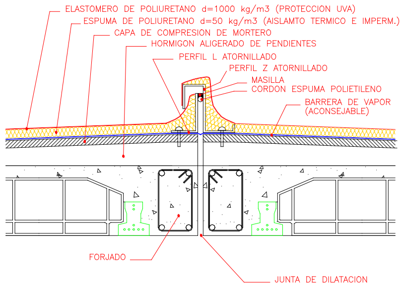
Detalle para salvar juntas de dilatación
